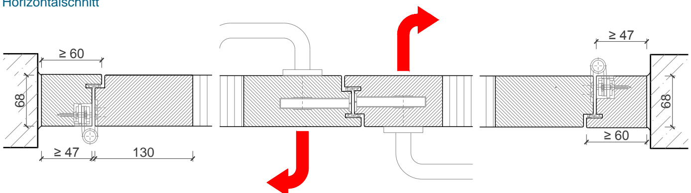
Horizontalschnitt
