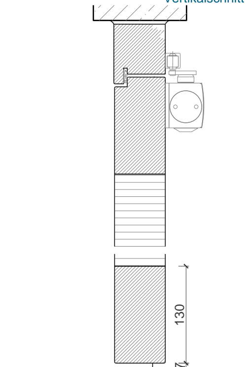
Vertikalschnitt
