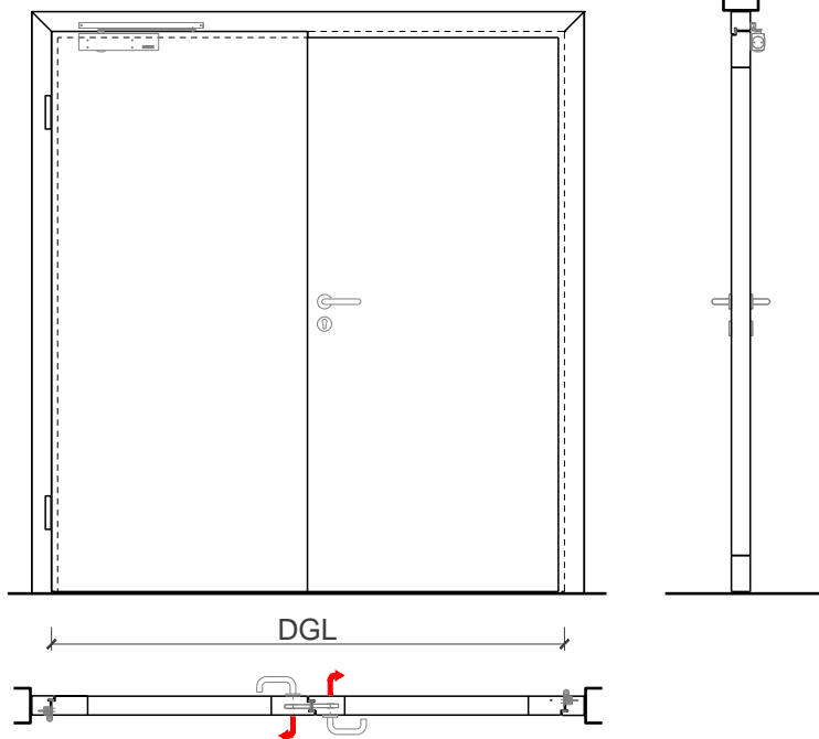
Horizontalschnitt
